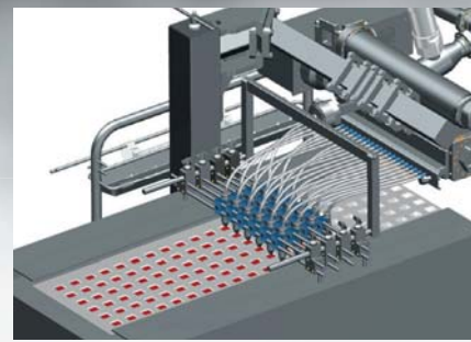
DS 552 para termoformadoras
